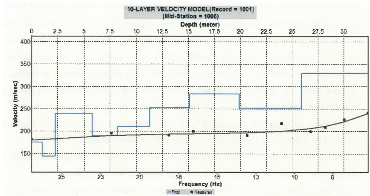
Fig. 8.2 – Profilo stratigrafico monodimensionale delle V_s .
