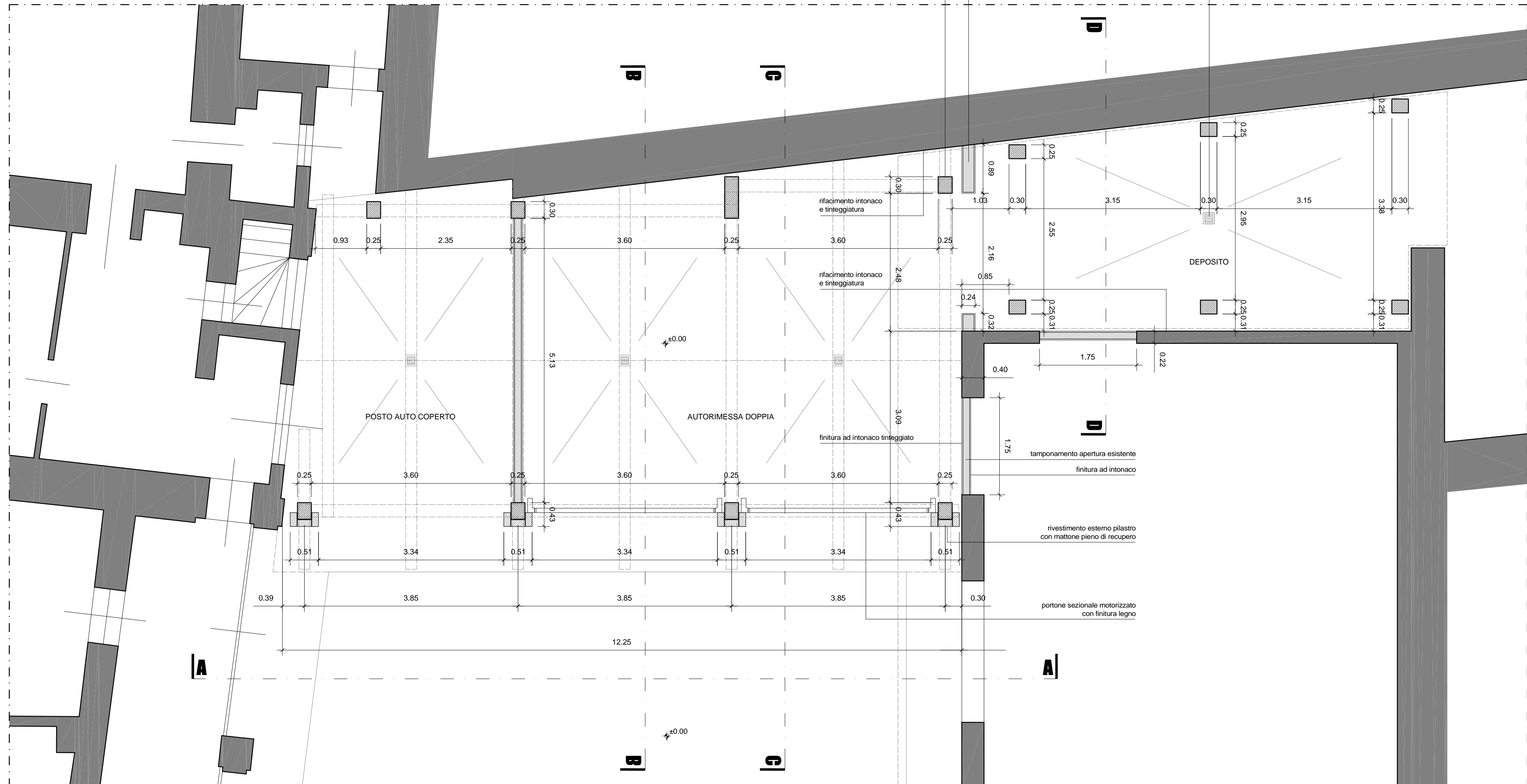
PIANTA - SCALA 1:50
