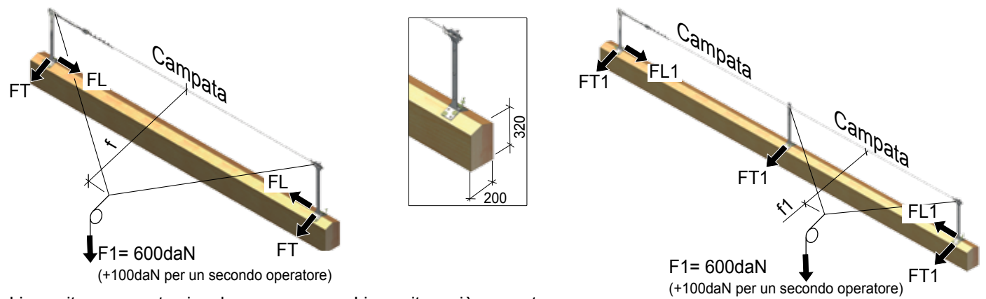
Linea vita a campata singola
