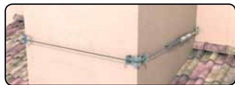
Caso di linea vita a parete su 3 lati: ancoraggi 601-601C come estremità e 601H-601L come intermedio.
